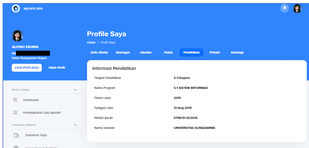
Gambar 7. Halaman Pendidikan
