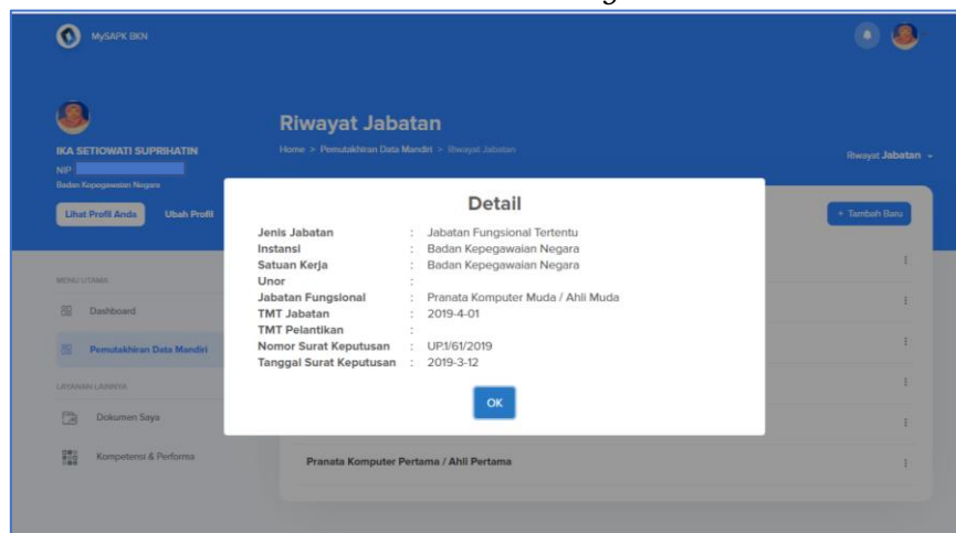
Gambar 47. Detail Jabatan
